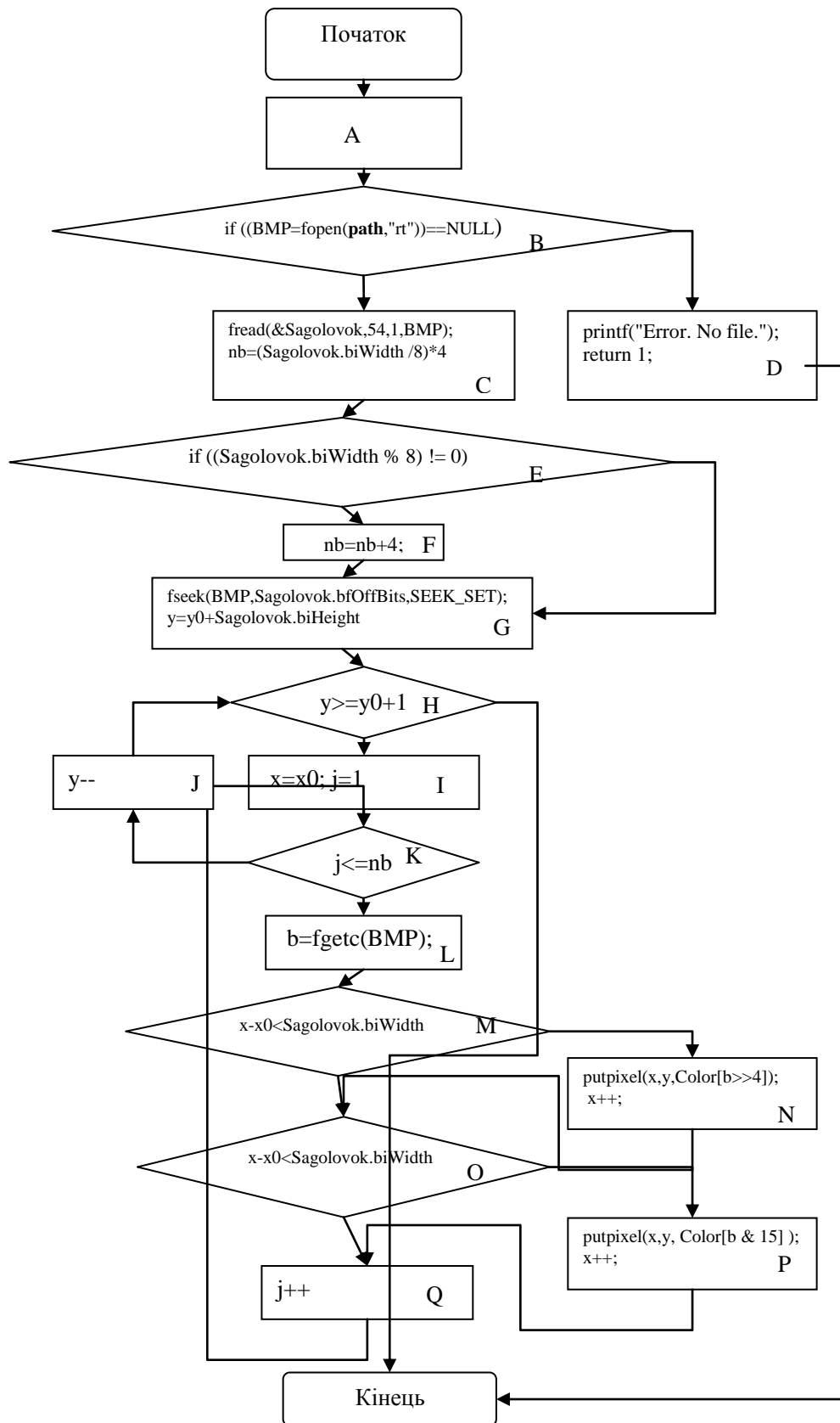
Рис. 2. Блок-схема програми.
